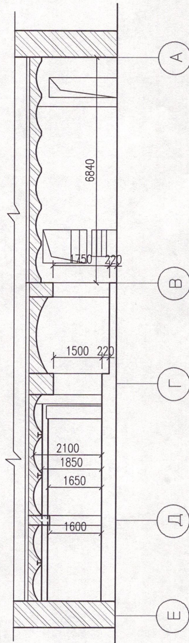
Розріз 1-1 (обмірний)
