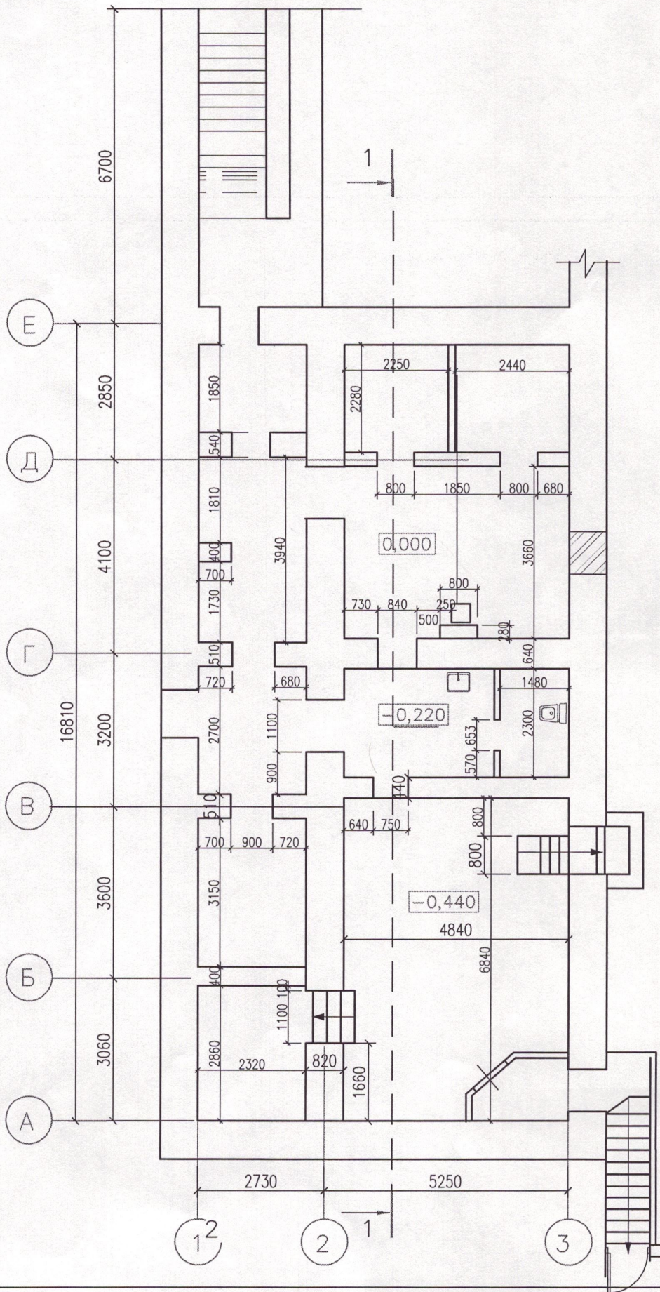
План підвальних приміщень (обмірний)
